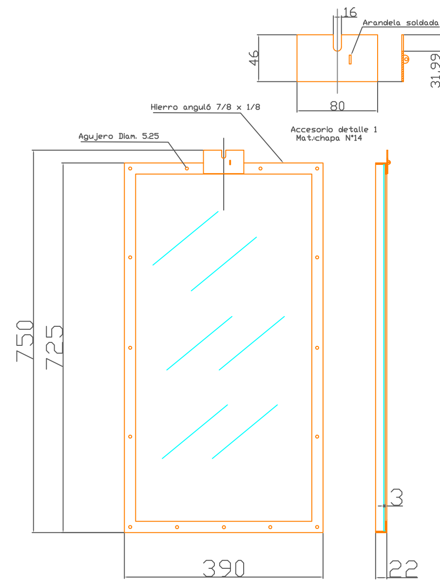
Contramarco para policarbonato 3 mm
