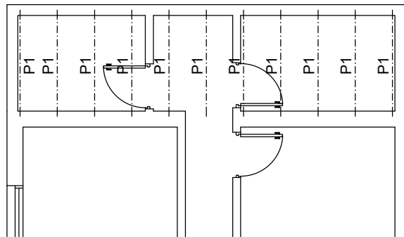
P1 - Perfil C80x50x15x2.00 galvanizado
